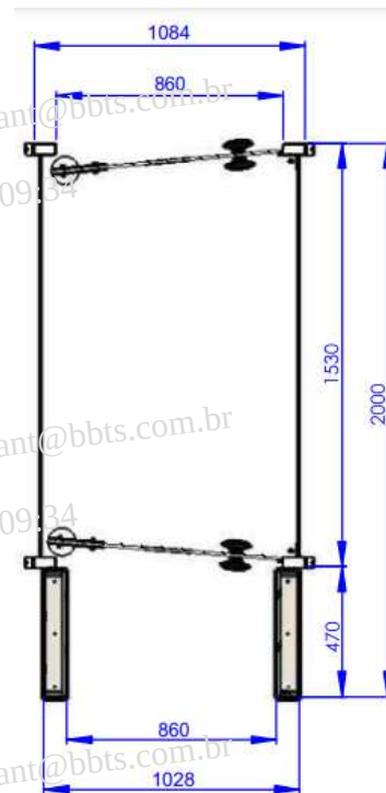
Imagem 04: PEDM modelos 1, 2, da tabela 03 acima.
